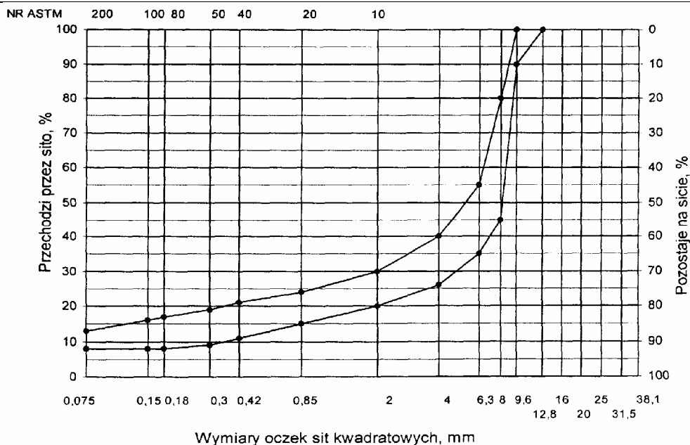
Rys. 5. Krzywe graniczne uziarnienia mieszanki mineralnej SMA od 0 do 9,6 mm do warstwy ścieralnej nawierzchni.
