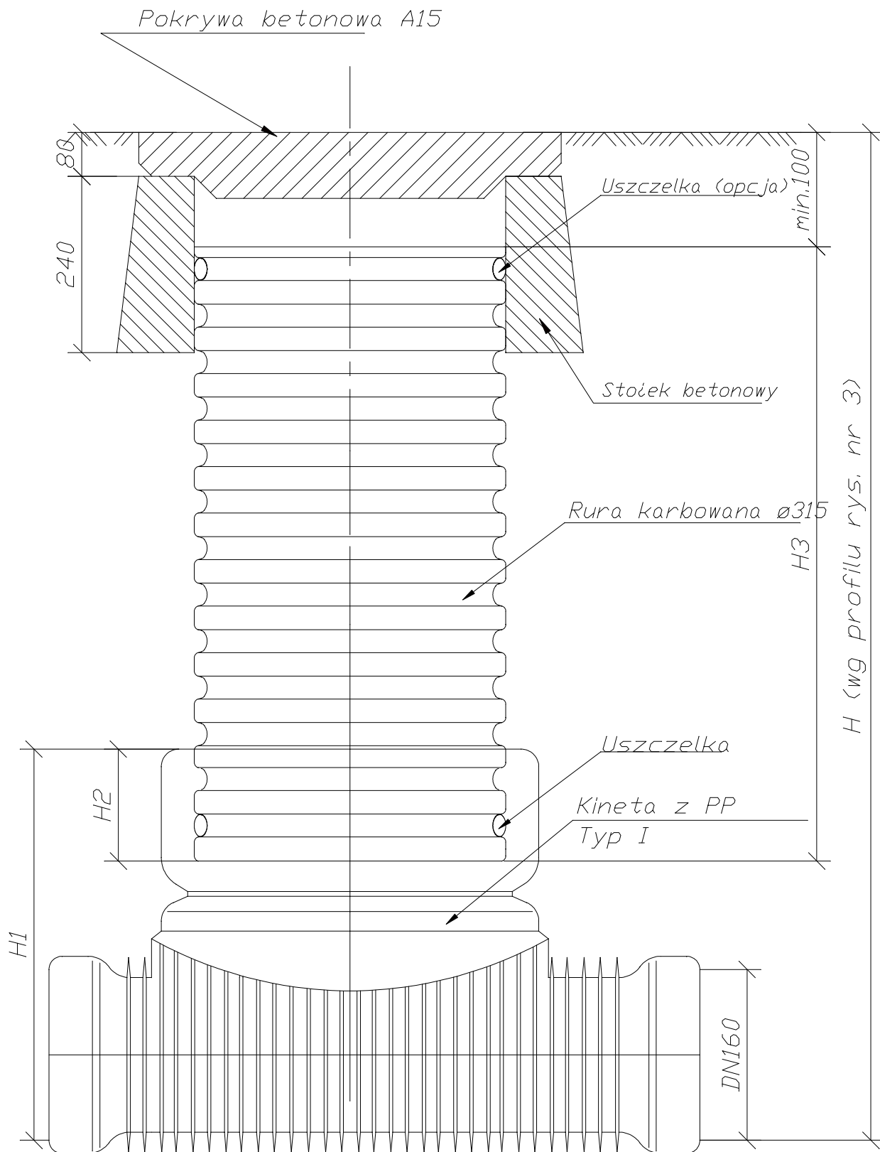
Studzienka kanalizacyjna ø315 niewłazowa
