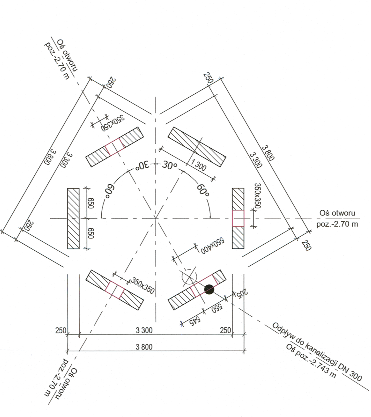
D-D 1:50
