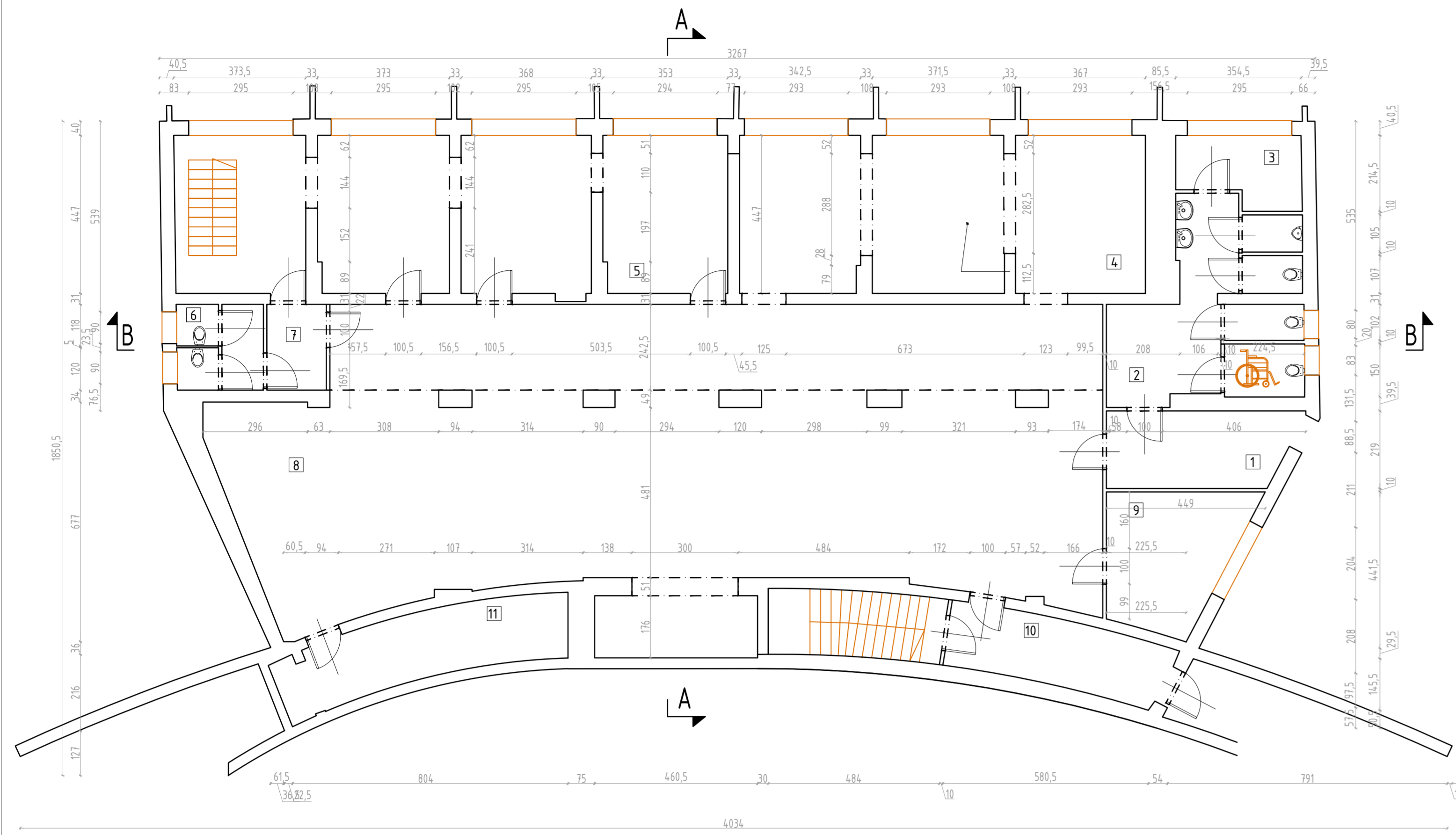
PARTER RZUT (+-0,00)
