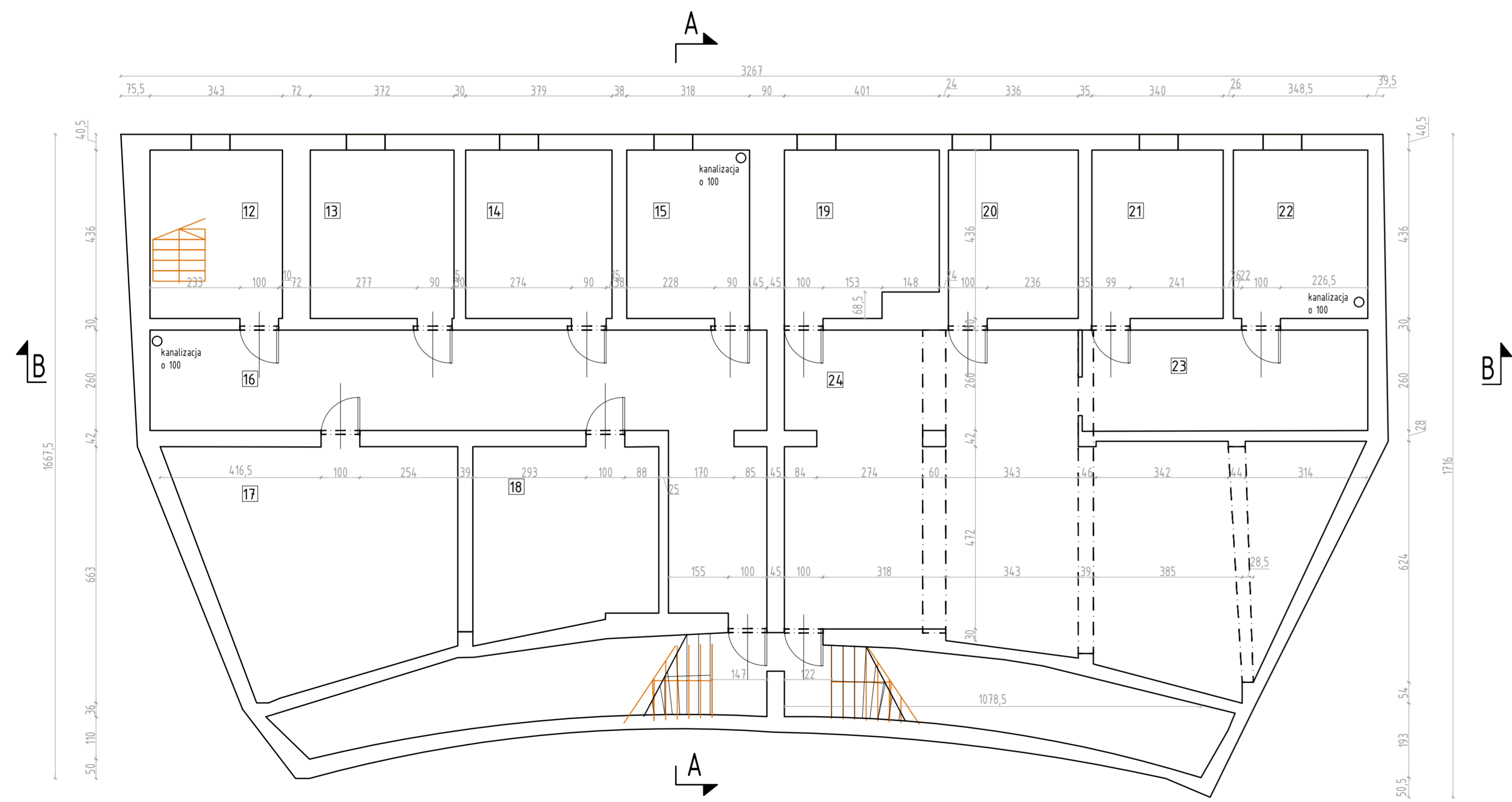
PIWNICE RZUT -2,75)
