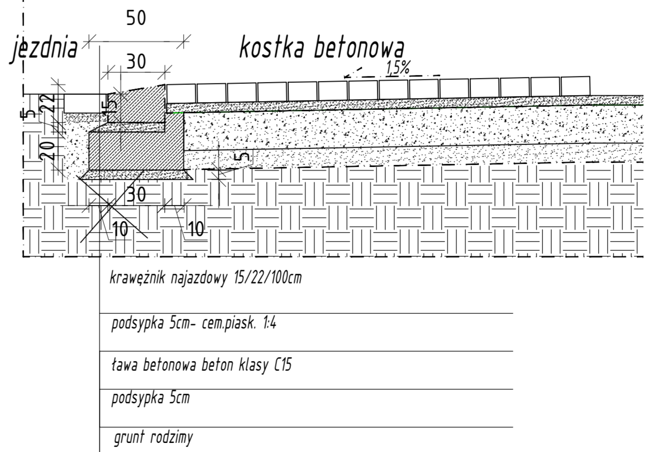
SZCZEGÓŁ B
