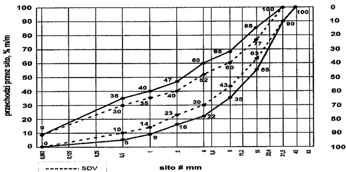
Rysunek 1. Uziarnienie mieszanki niezwiązanej 0/31,5 do w-wy podbudowy
